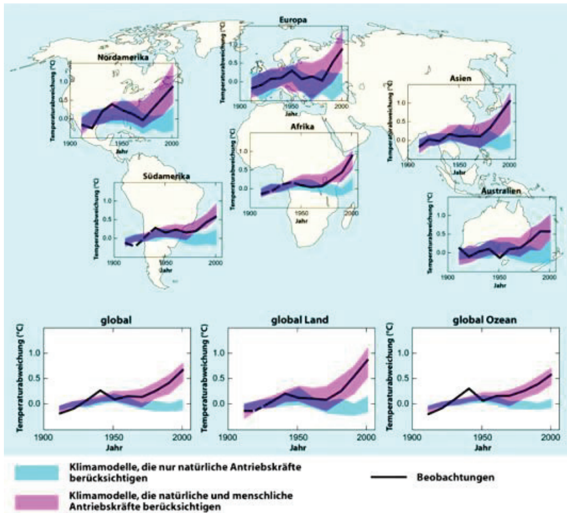
Abbildung 8: Globale und Kontinentale Temperaturveränderung (Quelle: IPCC, 2007a)
