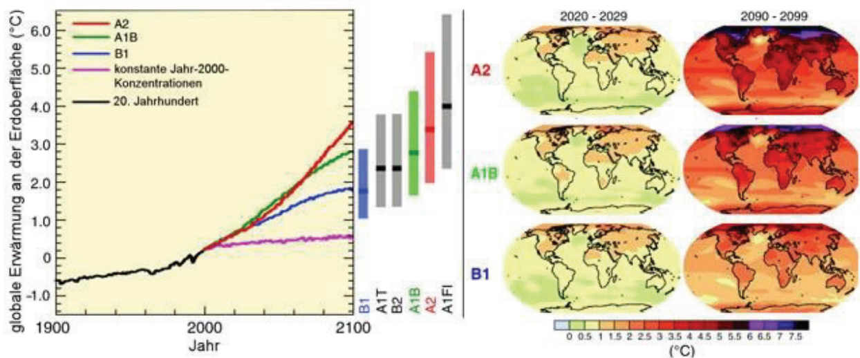
Abbildung 10: Entwicklung der Temperatur für 3 verschiedene Emissionsszenarien (Quelle: IPCC, 2007)
